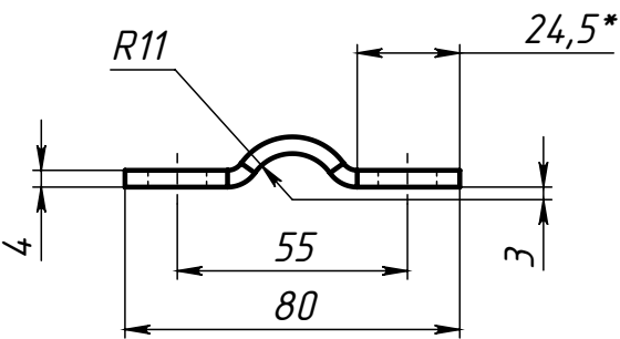
Поз.3 (Полухомут)
