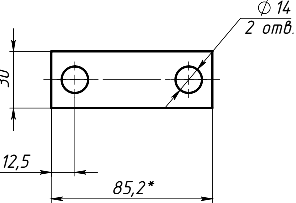
Поз.3 (Полухомут) развертка
